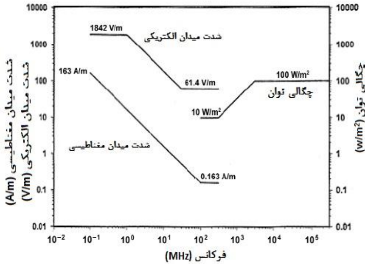
شکل ۵۲ - نمودار حد مجاز مواجهه شغلی امواج مایکروویو و رادیو فرکانسی (برای جذب ویژه تمام بدن کمتر از ۰/۴ W/kg)
